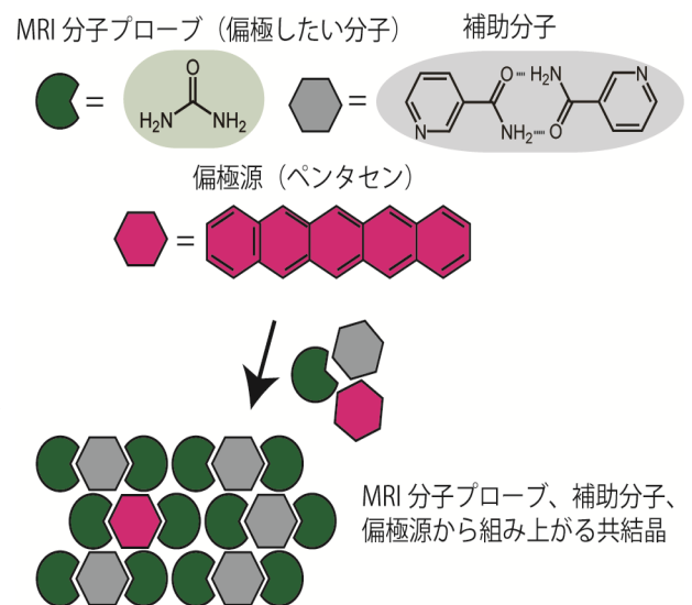
図 3. MRI 分子プローブなどのターゲット分子、補助分子、そして偏極源から組み上がる共結晶。
