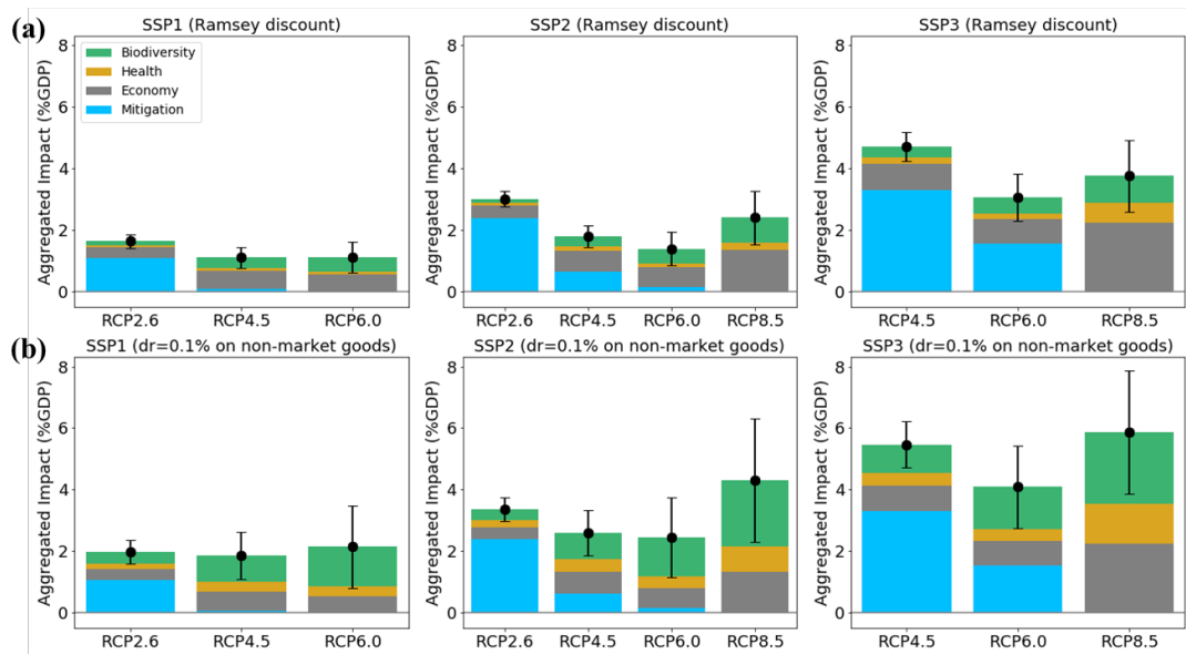
図 2：2010 年-2099 年の全世界について集計された気候変動の総費用。累積割引費用の累積割引 GDP に対する割合 (%)。(a)市場価値と非市場価値の両方に対してラムジー式に基づく割引率を適用した場合、および(b)市場価値はラムジー式に基づいた割引率、非市場価値は時間変化なしに 0.1%という割引率を適用した場合。点は平均値で、不確実性を示すバーは 5 つの GCM の結果間の 1 標準偏差。
