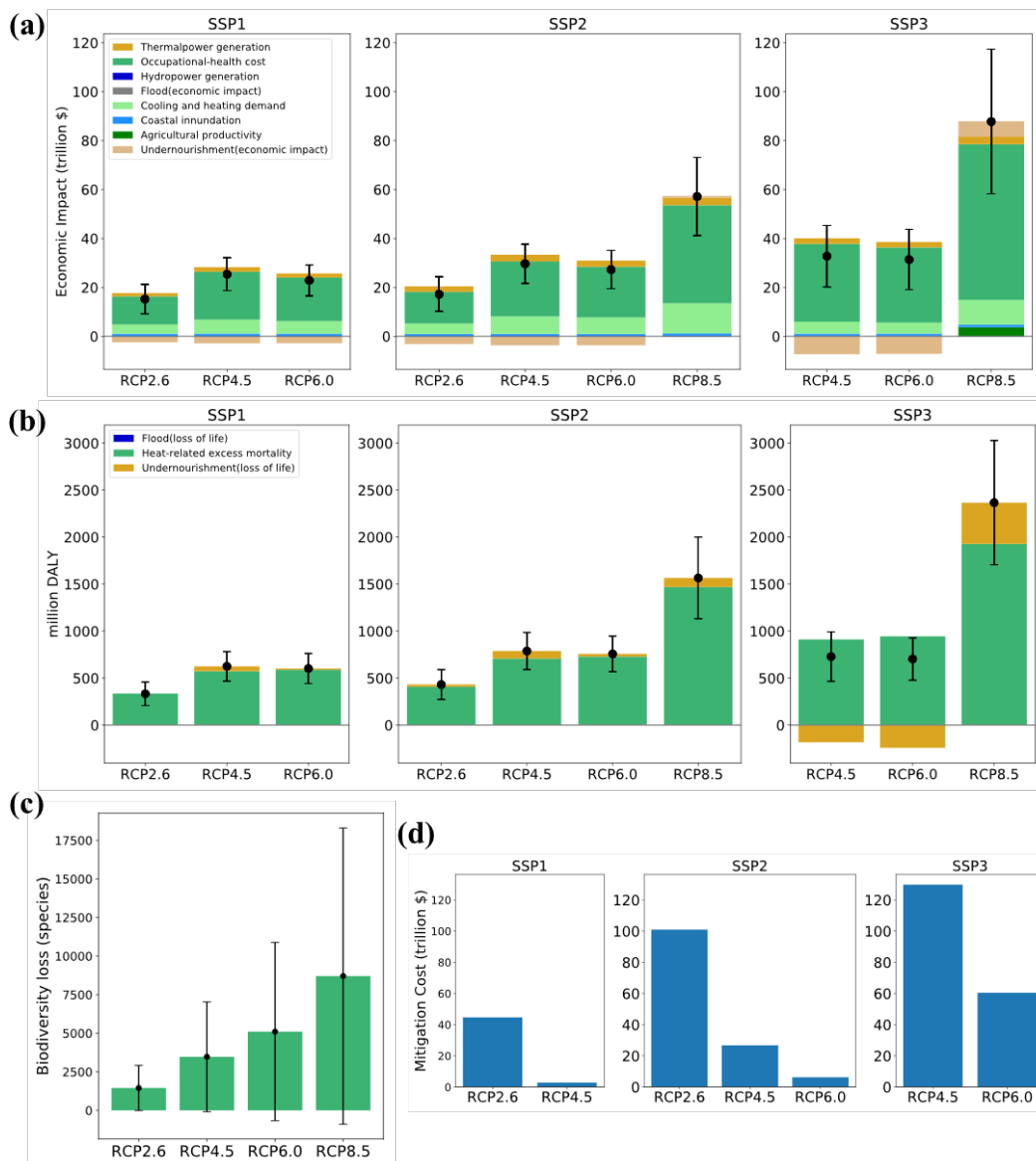
図1：3つの社会経済シナリオ(SSP)ごと、いくつかの温暖化レベル(RCP)ごとに推計された気候変動影響。(a)農業生産性、沿岸域の浸水、冷房と暖房の需要、河川洪水、水力発電、職業上の健康被害、火力発電、栄養不足という8つのリスク要因セクターにおける経済的影響、(b)人間健康(洪水や暑さに起因する過剰死亡率、および栄養不足)、(c)生物多様性、および(d)緩和費用。(a)と(d)の値は割り引かれた影響の累積値。SSP1/RCP8.5およびSSP3/RCP2.6を除きすべてのSSP1-3/RCP2.6-8.5の組み合わせに対する影響を棒グラフで示す。点は平均値、パーは5つの気候モデル(GFDL-ESM2M、HadGEM2-ES、IPSL-CM5A-LR、MIROC-ESM-CHEM、およびNorESM1-M)間の推計値の1標準偏差の不確実性。不確実性は、緩和費用以外のすべてのセクターについて考慮されている。(注：RCP：代表的な濃度経路。SSP：共有された社会経済的シナリオ。DALY：障害調整生存年数。)
