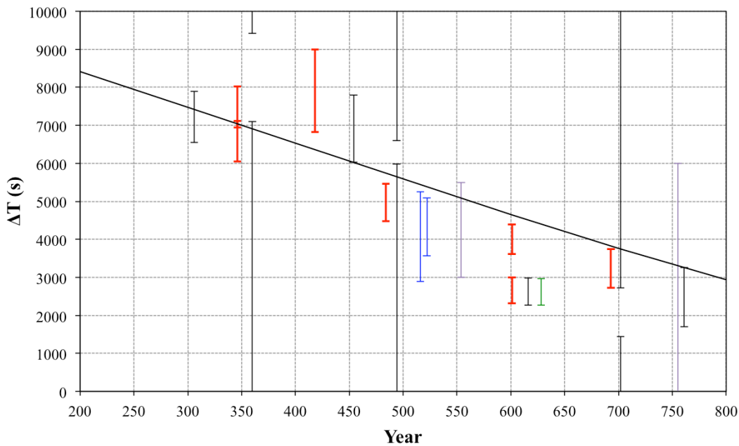
図3 西暦4世紀から7世紀ごろにかけての地球自転速度の変化 (Hayakawa, Murata, and Sōma 2022)。縦軸は \Delta T (上に凸のとき地球自転速度が速まり、下に凸のとき遅くなることを示す)、横軸は西暦年を示す。斜めに引かれた黒線は従来研究での地球自転速度変化の近似曲線。縦線は、皆既日食などの天文記録から算出された \Delta T の拘束幅を示し、黒、青、紫、緑が従来研究、赤が今回の検討で追加された地球自
