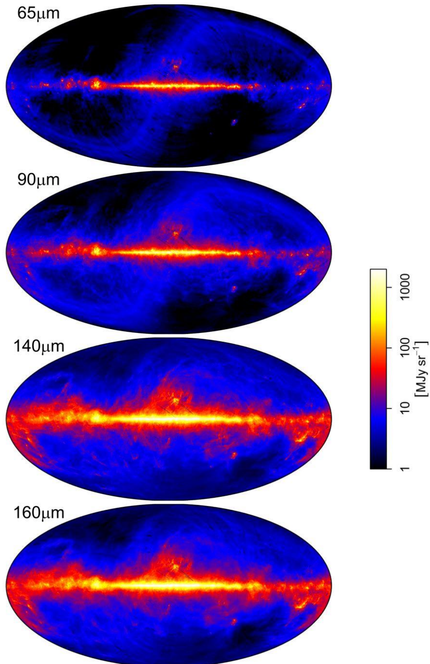
図 2 : 「あかり」は4つの波長で遠赤外線全天画像を作成した。図の上から順に 65 マイクロメートル、90 マイクロメートル、140 マイクロメートル、160 マイクロメートルの各全天画像を示す。中央に水平に伸びる天の川が各画像で明るく見える。一方、波長の長い画像は、より低温の星間物質の分布を示し、このような物質は天の川から上下方向により広がっていることが分かる。この差は 90 マイクロメートルと 140 マイクロメートルの 2 波長の画像の間で特に顕著である。100 マイクロメートルより短波長の 2 画像がこれまで「IRAS」により観測されていた遠赤外線の描像、一方 100 マイクロメートルより長波長の 2 画像が「あかり」が新しく描き出した遠赤外線の全天の詳細な分布である。
